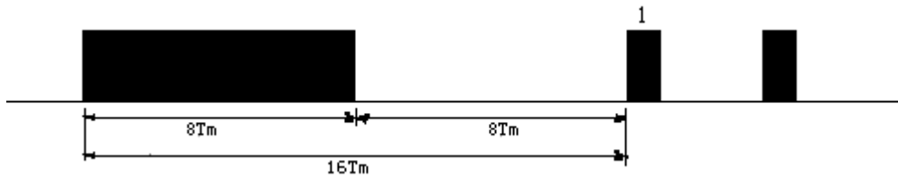
图3 TC9028-0E 的重复码波形
