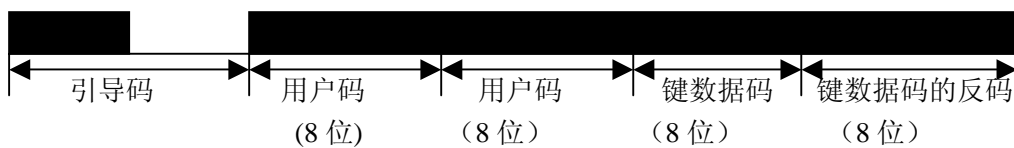
图 1 TC9028-0E 数据格式
