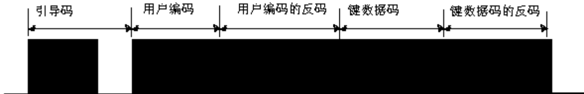
图 6 PT2222-14 数据格式
