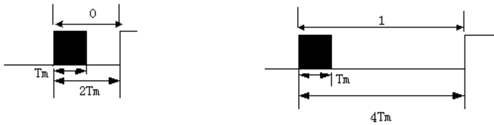
图4 TC9028-0E 的‘0’和‘1’的波形
