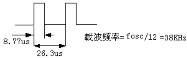
图5 TC9028-0E 的载波波形
