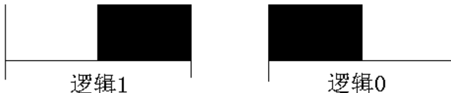
图 13 SAA3010-00 ‘1’ 和 ‘0’ 的波形
