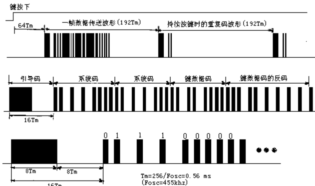
图 2 TC9028-0E 的发射波形
