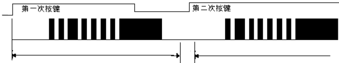
图 12 SAA3010-00 两次按键波形
