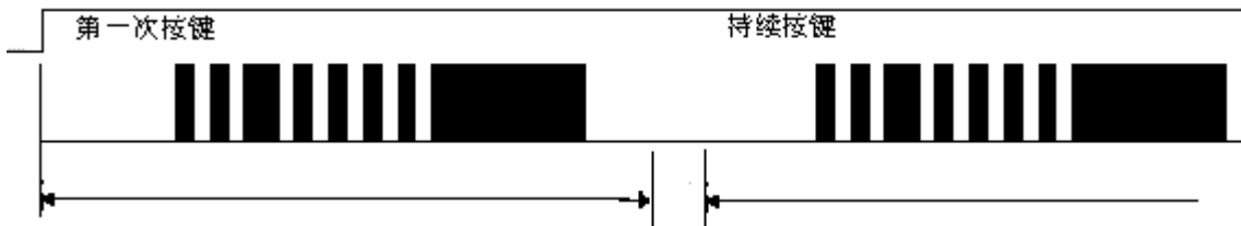
图 11 SAA3010-00 连续发射波形
