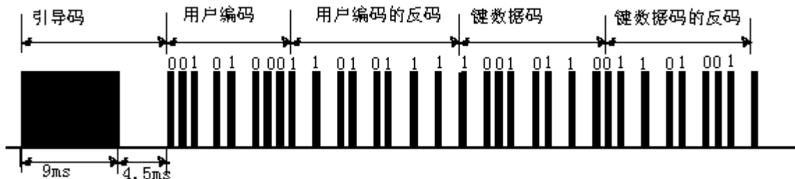
图 8 PT2222-14 的第一次传送波形
