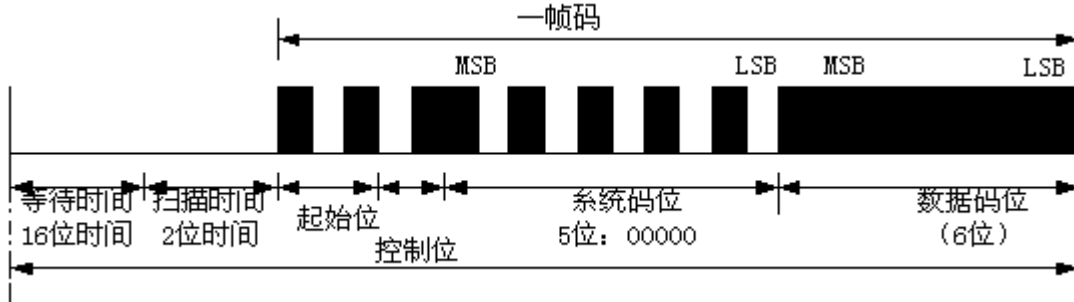
图 10 SAA3010-00 发射码波形
